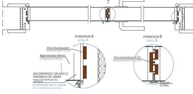
DUPLO ABRIR DOUBLE DOOR
