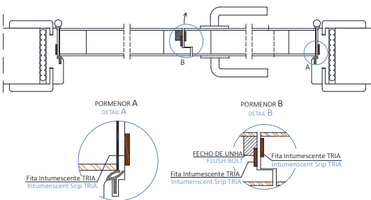
DUPLO ABRIR DOUBLE DOOR
