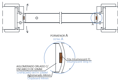
SIMPLES VAI-VEM DOUBLE ACTION SINGLE DOOR
