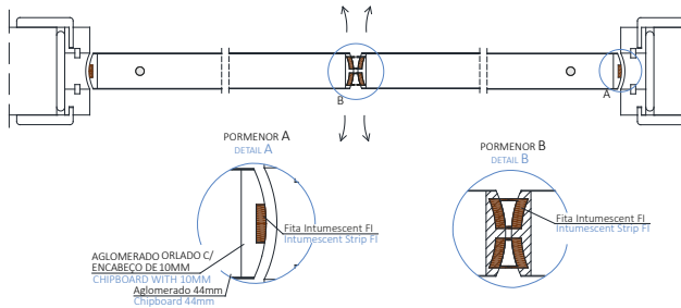
DUPLO VAI VEM DOUBLE ACTION DOUBLE DOOR
